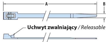
Zwalnialne Releasable
