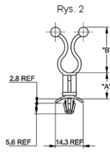
Wciskany w otwór: \varnothing 4.75 \pm 0.08 Grubość panelu: 0.8-2
