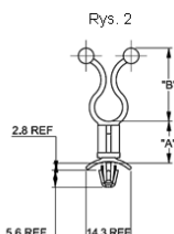
Wciskany w otwór: \varnothing 4.75 \pm 0.08 Grubość panelu: 0.8-2
