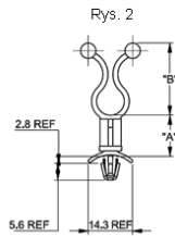
Wciskany w otwór: \varnothing 4.75 \pm 0.08 Grubość panelu: 0.8-2
