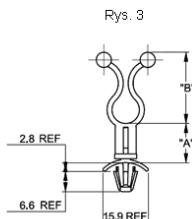
Wciskany w otwór: \varnothing 6 \pm 0.08 Grubość panelu: 0.78-2
