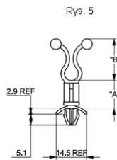
Wciskany w otwór: kwadrat 5.5 Grubość panelu: 0.8-2
