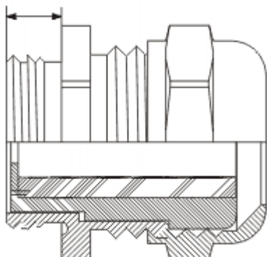
DŁUGOŚĆ GWINTU
