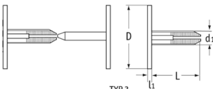
TYP 3
