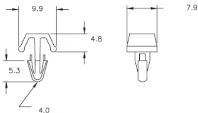
MB-156
