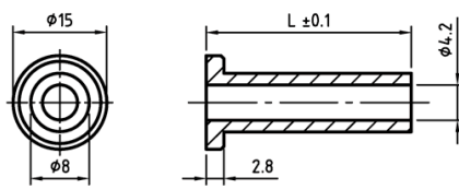
Typ 3 Type 3
