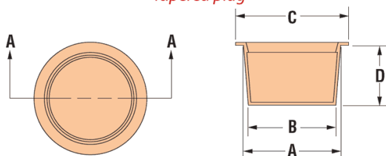
Zaślepka stożkowa Tapered plug
