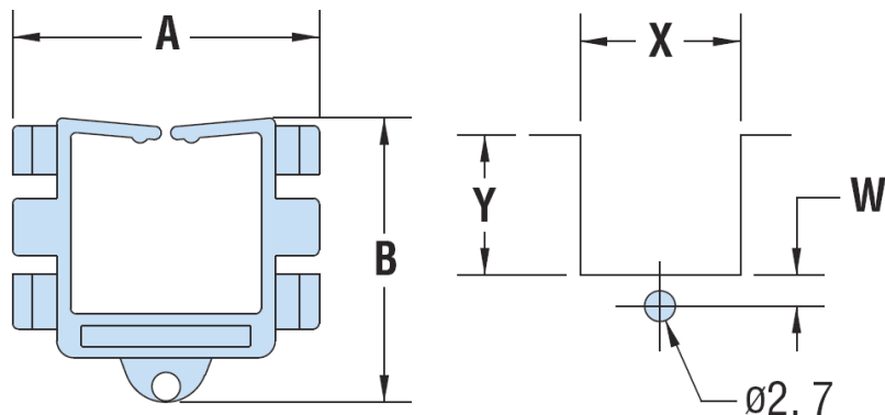
Wycięcie krawędziowe Edge slot
