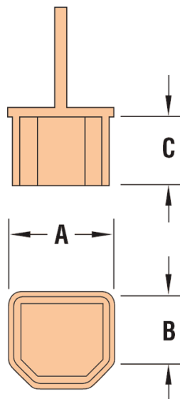
USB-B
