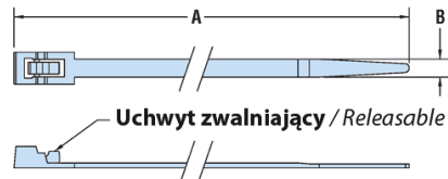
Zwalniające Releasable
