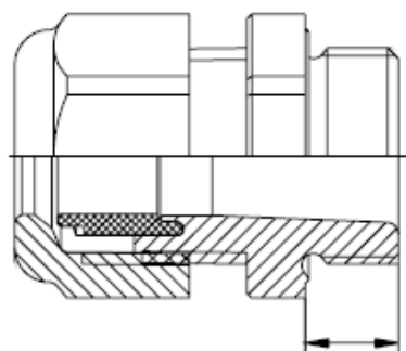
DŁUGOŚĆ GWINTU
