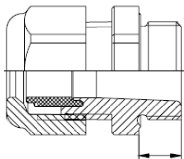
DŁUGOŚĆ GWINTU
