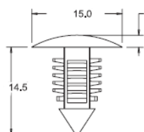
BPF-F2495
