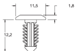
BPF-A414
