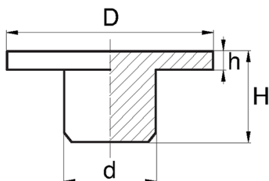
Typ 1 / Type 1
