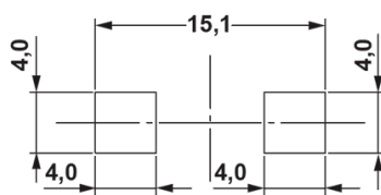
Otwór montażowy Typ 2 Type 2 Mounting hole
