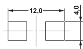
Otwór montażowy Typ 1 Type 1 Mounting hole
