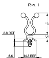
Wciskany w otwór: \square 4 \pm 0.08 Grubość panelu: 0.8-2
