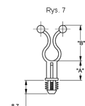
Rys. 7 Wciskany w otwór: \varnothing 7.9 \pm 0.08 Grubość panelu: minimum 6.4
