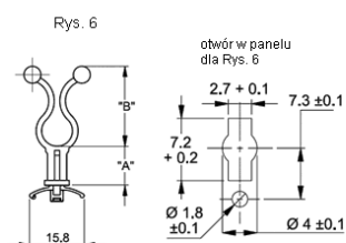
Rys. 6 Wciskany w otwór: jak na rysunku Grubość panelu: 0.8-1.6
