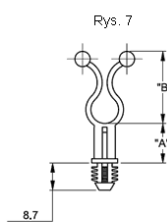
Rys. 7 Wciskany w otwór: \varnothing 7.9 \pm 0.08 Grubość panelu: minimum 6.4
