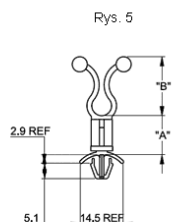
Wciskany w otwór: kwadrat 5.5 Grubość panelu: 0.8-2
