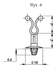
Rys. 4 Wciskany w otwór: \varnothing 6.5 \pm 0.09 Grubość panelu: 0.8-1.6
