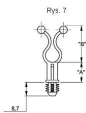
Wciskany w otwór: Ø7.9±0.08 Grubość panelu: minimum 6.4
