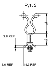
Wciskany w otwór: Ø4.75±0.08 Grubość panelu: 0.8-2
