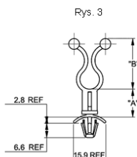
Wciskany w otwór: Ø6±0.08 Grubość panelu: 0.78-2
