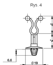
Wciskany w otwór: Ø6.5±0.09 Grubość panelu: 0.8-1.6
