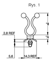
Wciskany w otwór: \varnothing 4 \pm 0.08 Grubość panelu: 0.8-2
