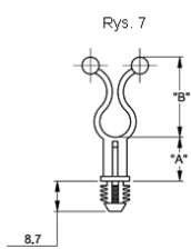
Wciskany w otwór: \text{Ø}7.9\pm0.08 Grubość panelu: minimum 6.4
