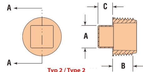
Typ 2 / Type 2
