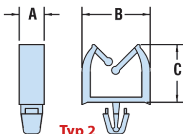
Typ 2 Type 2
