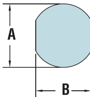
Sugerowany otwór Suggested clearance hole
