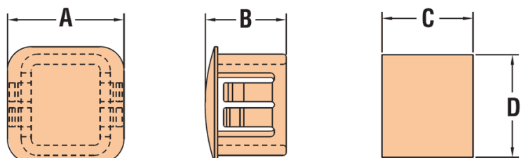
Otwór montażowy Mounting hole
