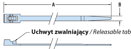
Zwalniające Releasable
