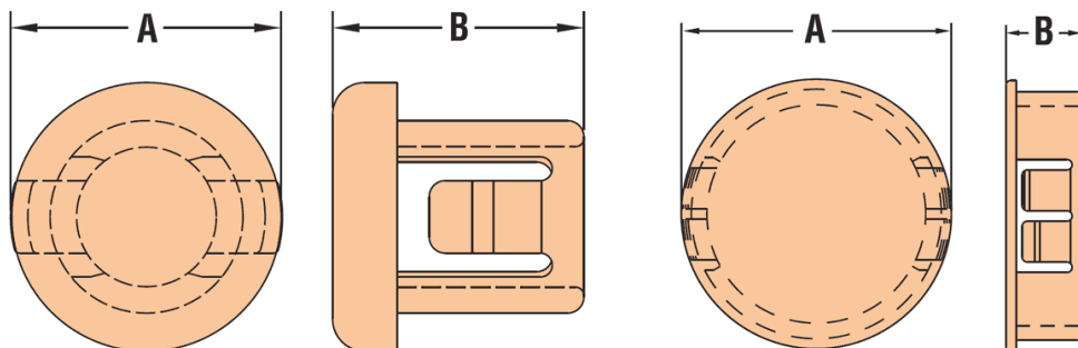
Dla pojedynczej grubości panelu Single panel thickness design
