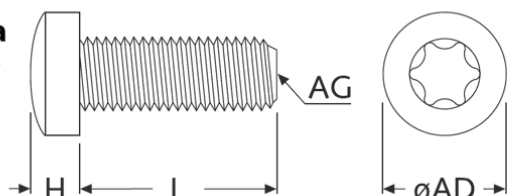
Śruba Screw
