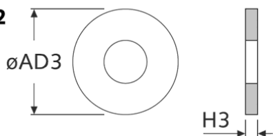
Podkładka 2 Washer 2
