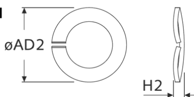
Podkładka 1 Washer 1
