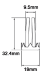
Typ 5 metalowe gniazdo na trzpień zatraskowy
