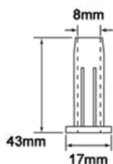
Typ 4 plastikowe gniazdo na trzpień zatraskowy
