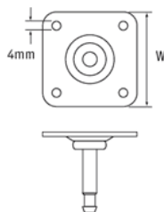
Typ 3 mocowanie płytkowe
