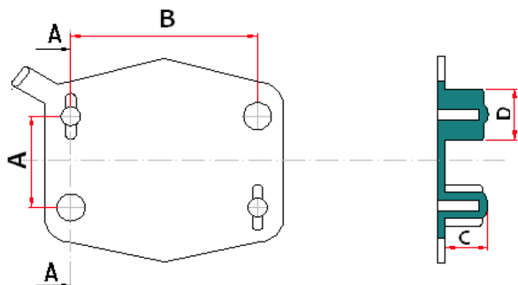
SEZ. A:A
