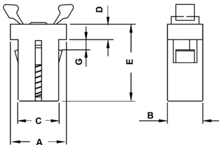
4715GA01PS
