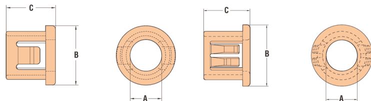
Typ 1 - pojedynczy panel Type 1 - single panel design
