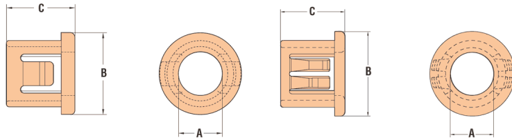
Typ 1 - pojedynczy panel Type 1 - single panel design
