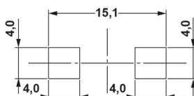
Otwór montażowy Typ 2 Type 2 Mounting hole
