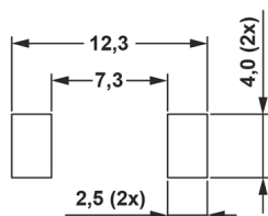
Otwory montażowe Mounting holes
