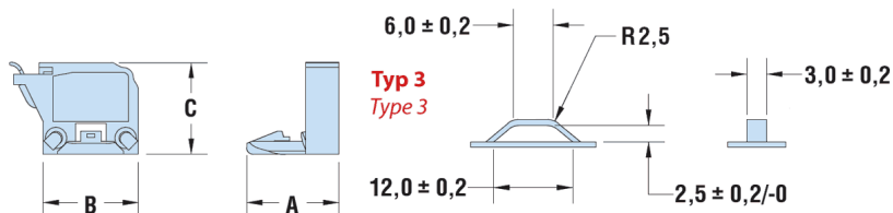
Wymiary otworu montażowego Mounting hole dimensions
