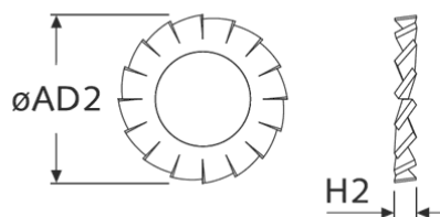
Podkładka 1 Washer 1
