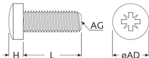
Śruba Screw
