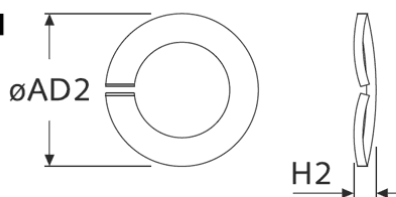
Podkładka 1 Washer 1
