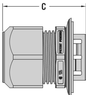
Uszczelka / kołnierz uszczelniający Sealing flange/washer construction
