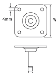
Typ 3 mocowanie płytkowe
