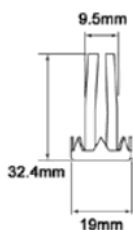
Typ 5 metalowe gniazdo na trzczeń zatrzaskowy
