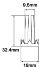
Typ 5 metalowe gniazdo na trzczeń zatrzaskowy
