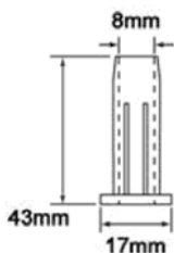
Typ 4 plastikowe gniazdo na trzczeń zatrzaskowy
